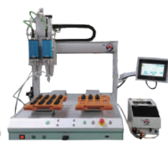
SR-雙伺服電批鎖螺絲機
