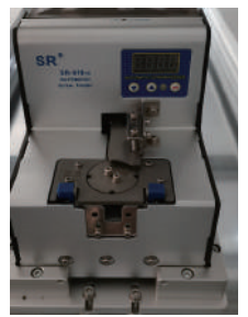
吸附式供料器 Adsorption feeder
