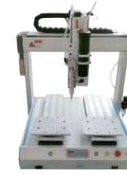
SR-自動點膠機
